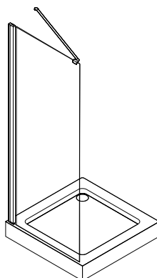
Seitenwand schließseitig 1 × CSW1590 (Breite 900 mm)
